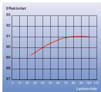
MISSION™ 3-Pass har en virkningsgrad på 91% ved fuld belastning - og holder en høj effektivitet i hele lastområdet. Hvis anlægget forsynes med økonomiser, kan virkningsgraden øges til 95%.
